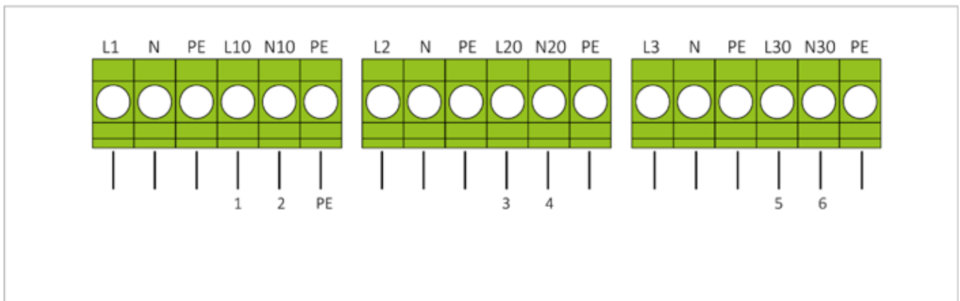
Abb. 10: Anschlussfeld in der Leistungselektronik
