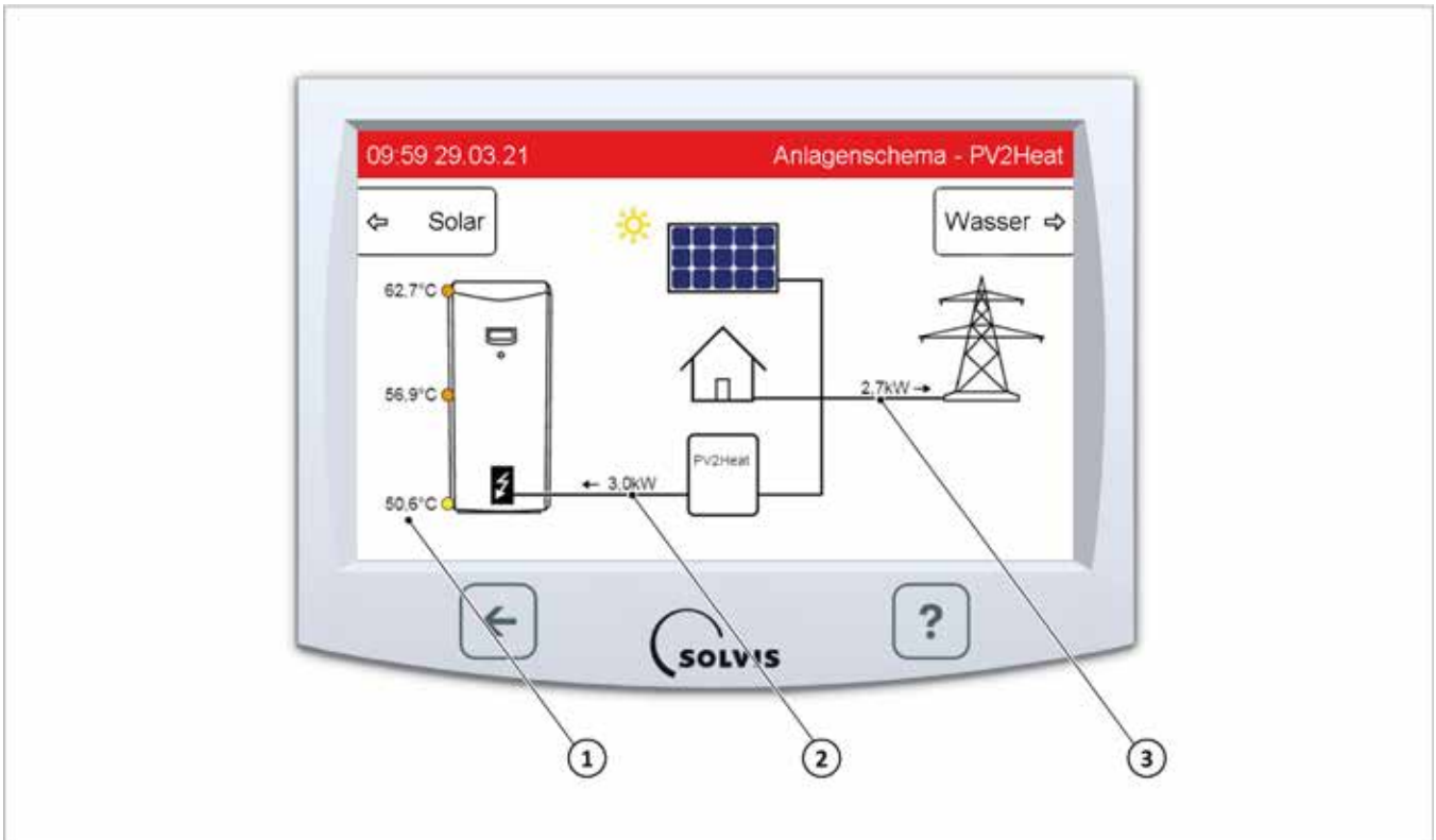
Abb. 18: AnlagenschemaSolvisPV2Heat SC-3
