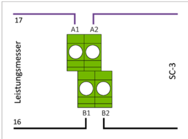
Abb. 15: Modbus-Anschluss in der Leistungselektronik (6kW)
