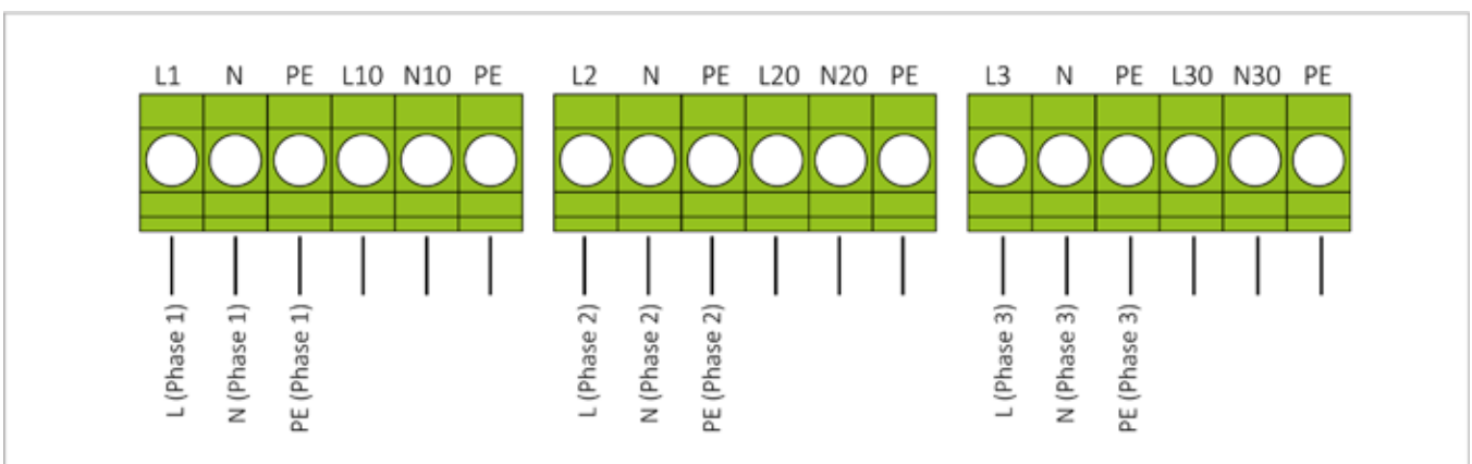
Abb. 14: Anschlüsse der Spannungsversorgung
