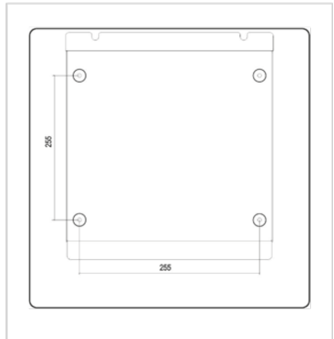
Abb. 9: Maße für Bohrlöcher
