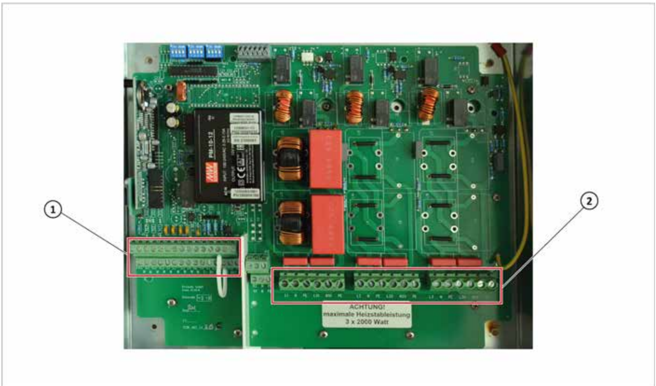
Abb. 13: Anschlüsse auf der Platine der Leistungselektronik
